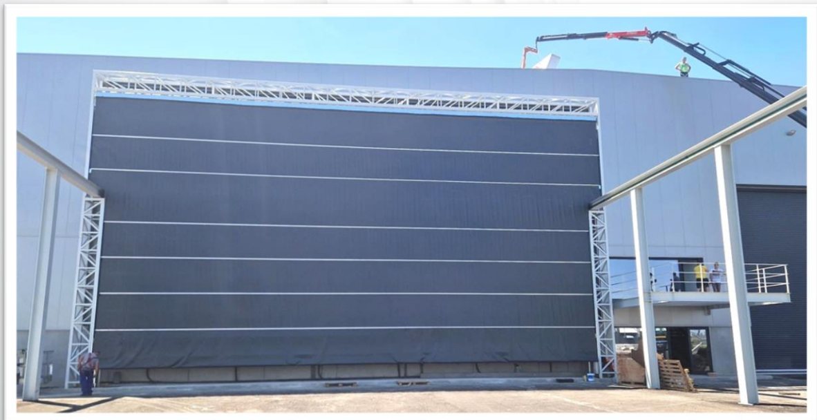
Versione Mega Pack L. 25 x H. 16 mt.
