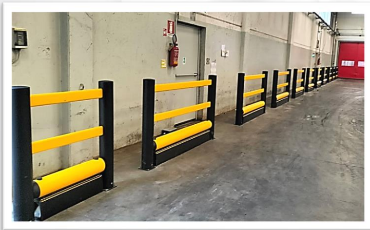
Soluzione per corsie pedonali
