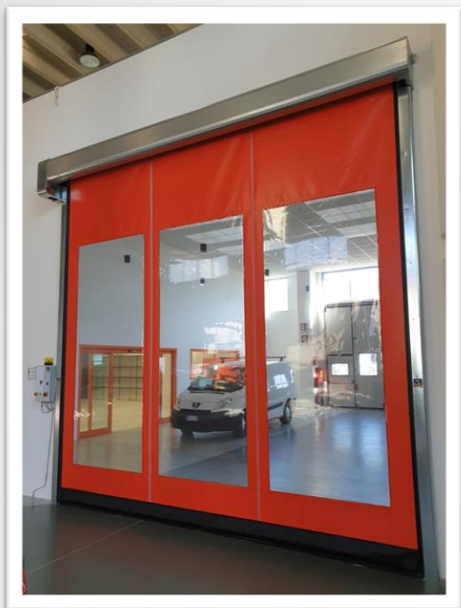
Esecuzione con manto Full Vision
